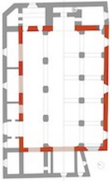
Floor plan of the Seville's synagogues. Oscar Gil Delgado. "Una sinagoga desvelada en Sevilla: estudio arquitectónico". Sefarad 73 (2013), p. 92.
