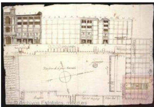
Traza del plano de situación y alzado de las casas y tiendas de la plaza de Bibarrambra (Floorplan of Bibarrambra square, 1616)
