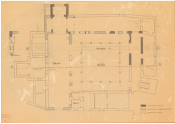
Alhambra. Convento de San Francisco. Planta baja y sección (con anotaciones arqueológicas) [1927-1928]
