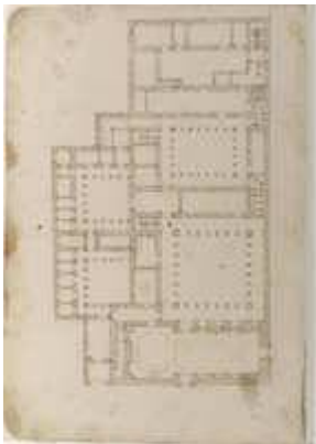
Planta del convento de Nuestra Señora de la Merced de Sevilla
